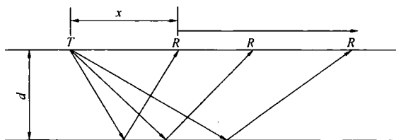
图 1 宽角法示意
