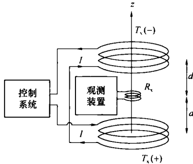
图 22 等值反磁通装置示意
