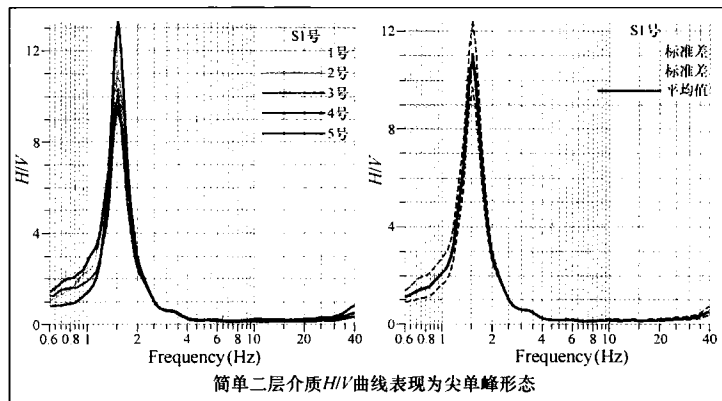
图 17 简单二层介质 H/V 曲线
