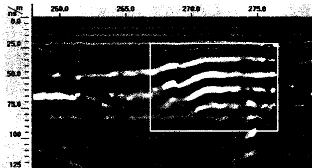
图 15 地下工程加固体（注浆）
