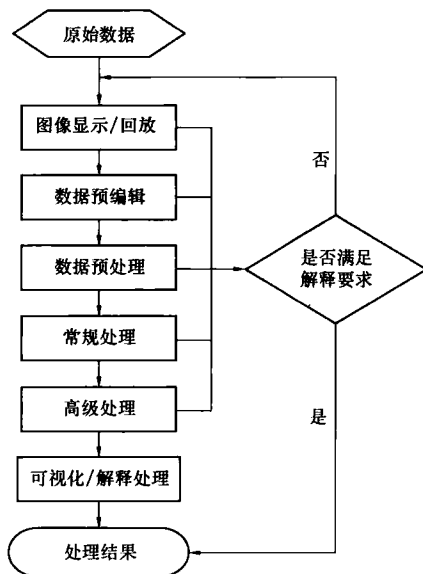
图 6.2.15 探地雷达数据处理流程
