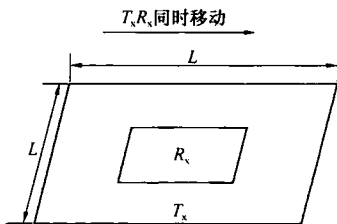
图 21 中心回线装置示意
