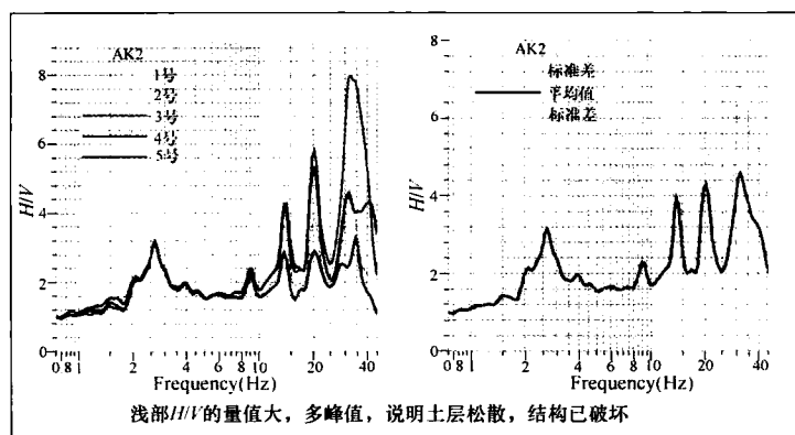
图 19 疏松体 H/V 曲线
