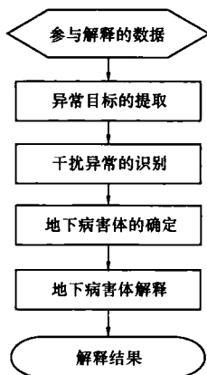
图 6.2.17 探地雷达法资料解释流程
