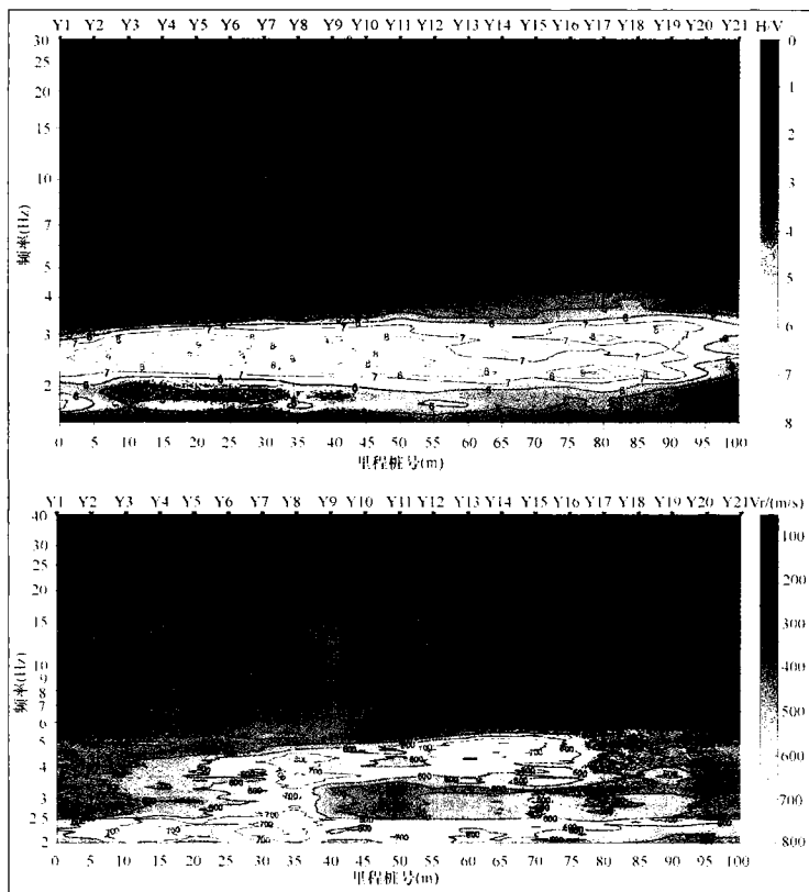
图 20 疏松体的 HV 曲线剖面 (上图) 与相速度剖面 (下图) 对比
