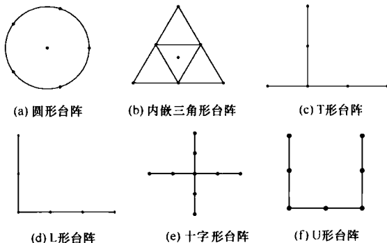
图 16 微动勘探法台阵布设方式示意
