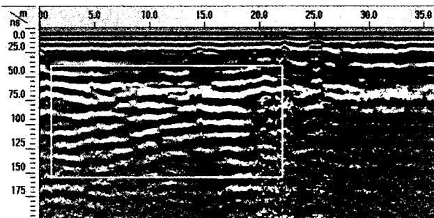
图 6 金属围挡
